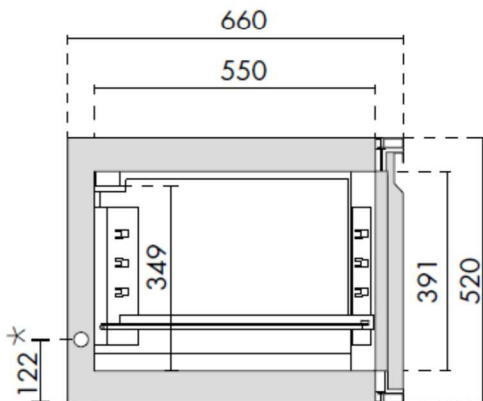
Ansicht Kühlpult mit Flügeltür
