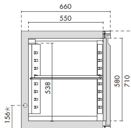
Ansicht Kühlpult mit Flügeltür
