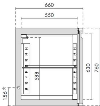
Ansicht Kühltisch mit Flügeltür
