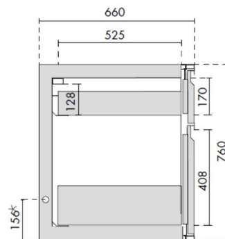
Ansicht Kühltisch mit Lade 1/3 - 2/3
