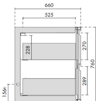
Ansicht Kühltisch mit Lade 1/2 - 1/2
