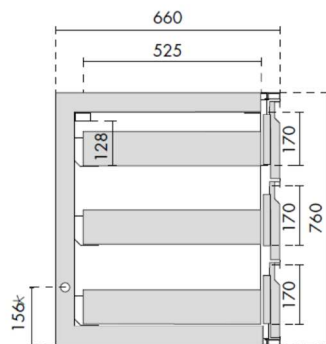
Ansicht Kühltisch mit Lade 1/3 - 1/3 - 1/3
